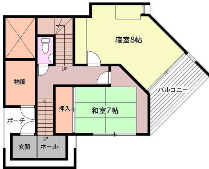
1階平面図
